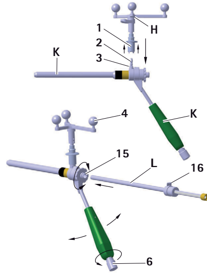
Şekil 12 Aesculap yıldız ünitesinin S 4 C kılavuz kovan üzerine montajı; S 4 C iç delme kovani üzerine yerleştirilmesi
