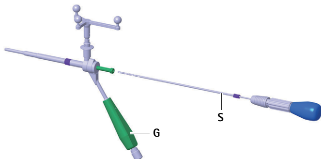
Fig. 4 Violett markering på S 4 C-navigerad bormall och borrar
