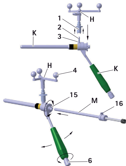
Fig. 13 Montaggio dell'unità a stella Aesculap sulla bussola guida S 4 C; inserimento del calibro di foratura S 4 C
