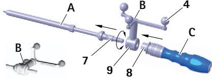
Şekil 6 Referans yıldız ünitesi ekipmanının ("pre-calibrated") ve S 4 C el tutamağının S 4 C dişli kesicisine montajı
