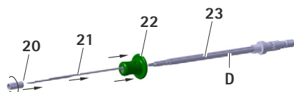
Obr. 20 Montáž skrutkovača S 4 C
