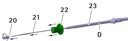
Fig. 15 Démontage du tournevis S 4 C
