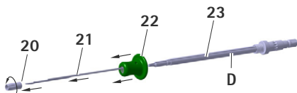
Fig. 15 Demontering S 4 C-skruvmejsel
