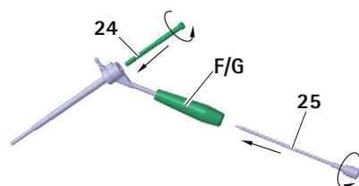
Obr. 21 Montáž vrtacieho kalibru S 4 C
