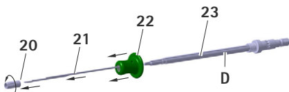
Abb. 15 Demontage S 4 C-Schraubendreher
