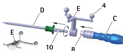
Fig. 8 Montaje del instrumento de la unidad en estrella de referencia (calibración con ICM 4) y del mango S 4 C (FW067R o FW165R) en el destornillador S 4 C
