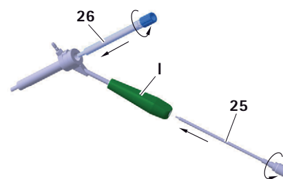
Obr. 22 Montáž vodiaceho puzdra pre skrutky s hladkým dříkom
