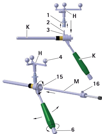
Fig. 13 Montering av Aesculap-stjärnenheten på S 4 C-styrhylsan; insättning av S 4 C-borrmallen
