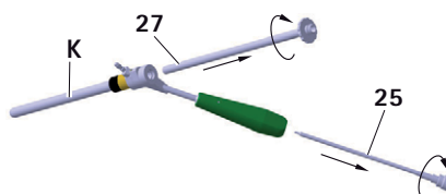
Fig. 18 Desmontaje del casquillo de guía Ø 3,5 mm/4,0 mm
