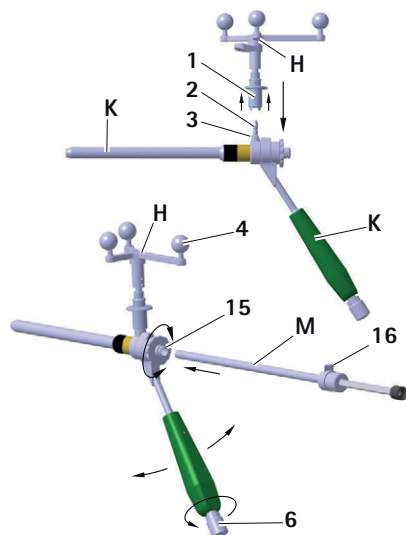
Afb. 13 Montage van de Aesculap-stereenheid op de S 4 -geleidingshuls; plaatsen van de S 4 -boormal
