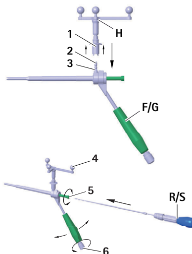
Fig. 5 Montaje de la unidad en estrella Aesculap sobre la guía S 4 C FW664R/FW665R
