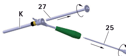
Rys. 18 Demontaż tulejki prowadzącej Ø 3,5 mm/4,0 mm
