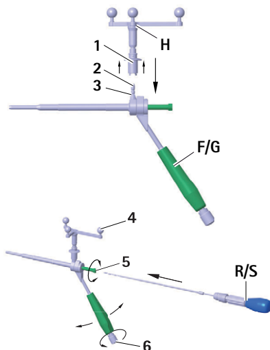
Fig. 5 Montaggio dell'unità a stella Aesculap nel calibro di foratura S 4 C FW664R/FW665R
