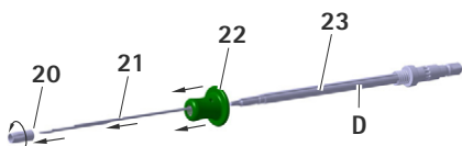
Obr. 15 Demontáž skrutkovača S 4 C
