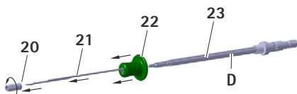
Fig. 15 Desmontagem da chave de fendas S 4 C
