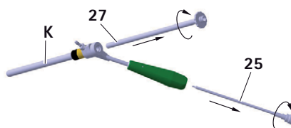
Obr. 18 Demontáž vodící objímky Ø 3,5 mm/4,0 mm
