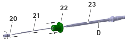
Рис. 20 Монтаж отвертки S 4 C
