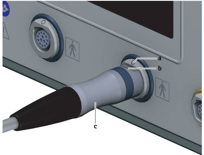
Abb. 3 Motorkabel anschließen
